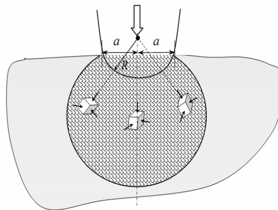
Рис. 4. Контакт тупого індентора з еластопластическим напівпростором: штрихувкою позначена зона трохосного рівномесного стиснення
